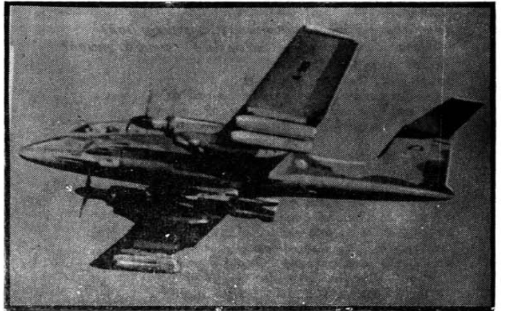
புக்காரா : மணிக்கு 500 கி. மீ. வேகம்; 1500 கி. கி. நிறையுடைய 1A 58A Pucara குண்டுகளை எடுத்துச் செல்லும்.
