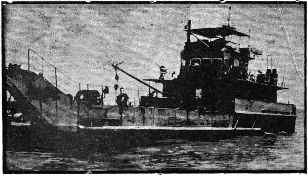
ஒரே தடவையில் சுமார் 600 படைவீரர்களைக் கொண்டுசென்று தரையிறக்கக்கூடிய இந்தக்கலம், கடற்கரை வந்து (1 அடி தண்ணீரில்) படையினரை இறக்கிவிடக்கூடியது. இவ்வகைக் கலங்கள் நான்கு தற்போது சிங்களக் கடற்படையிடம் உண்டு.
