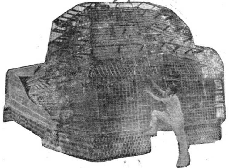
ஒரு கவச வாகனம்போல் எம்மால் தயாரிக்கப்பட்ட "புல்டோசர்" வண்டி.
